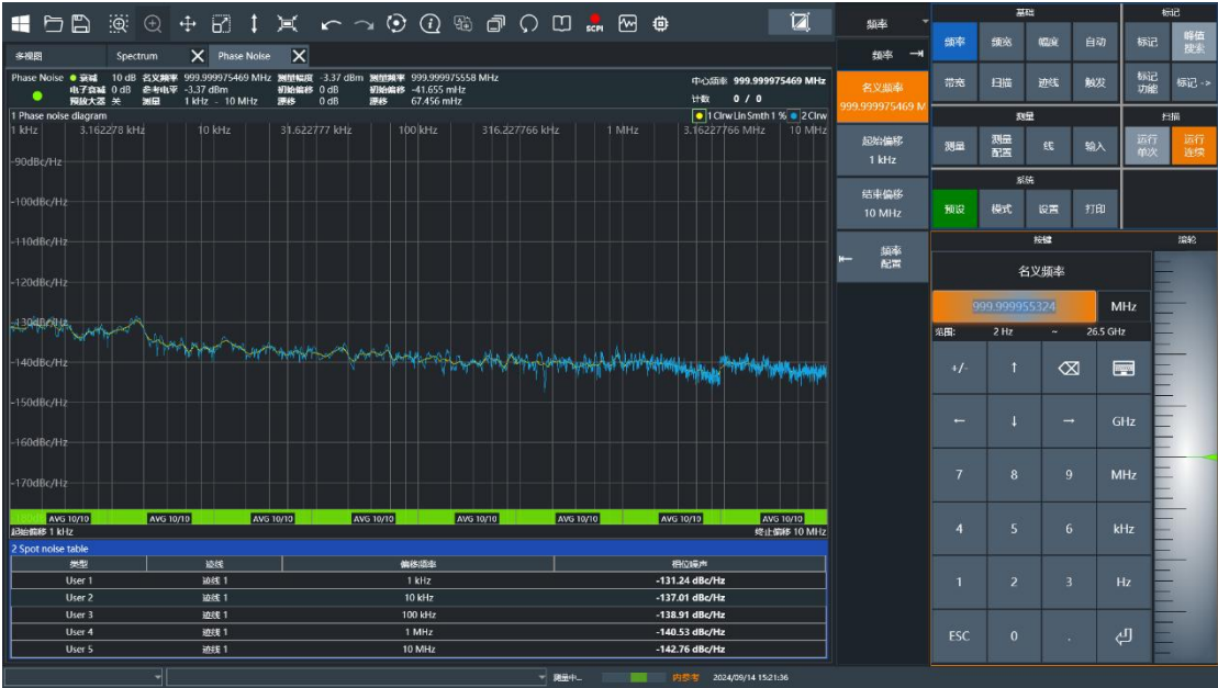
相位噪声实测界面
