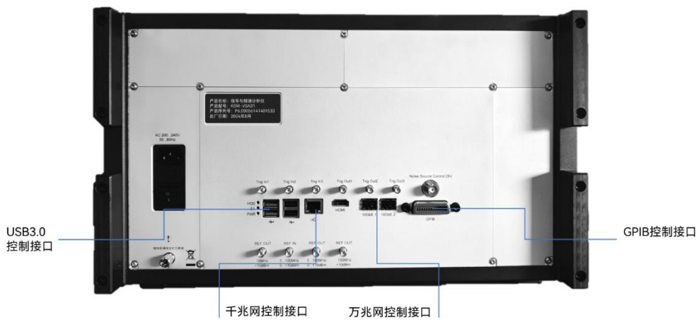
背面板接口图
